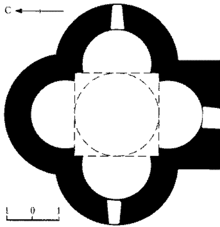
План ц. Аствацацин мон-ря Прцив (Армения). Сер. VII; XII в.
